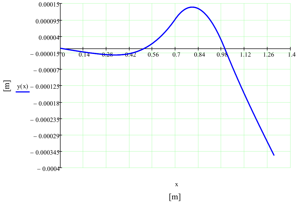
Verlauf der Durchbiegung am gesamten Träger
