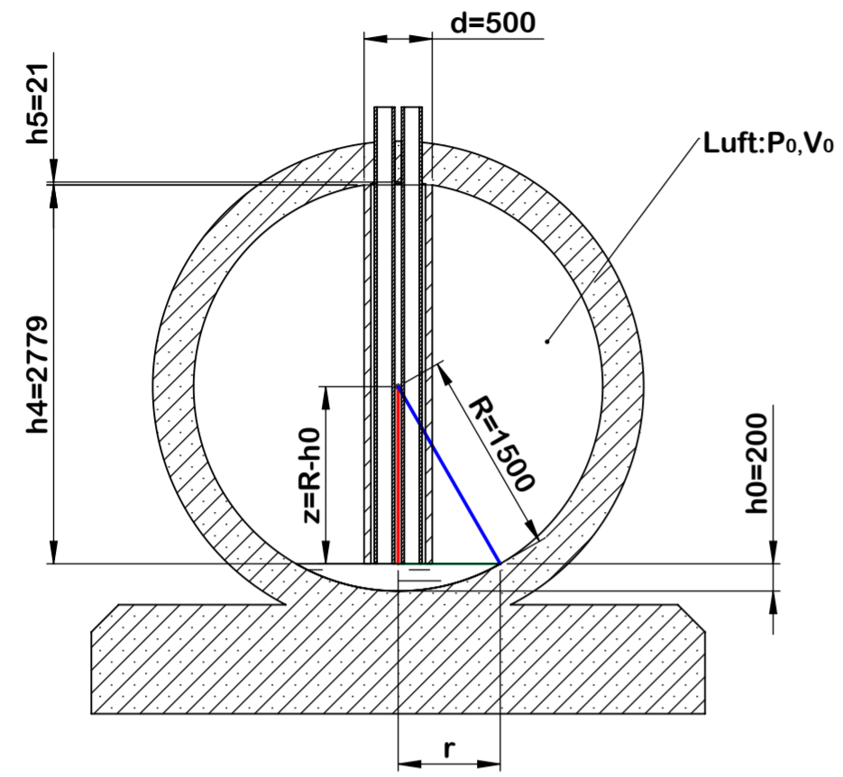
SCHNITT A-A
