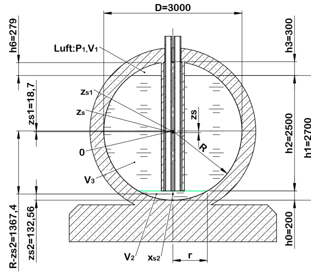
SCHNITT B-B
