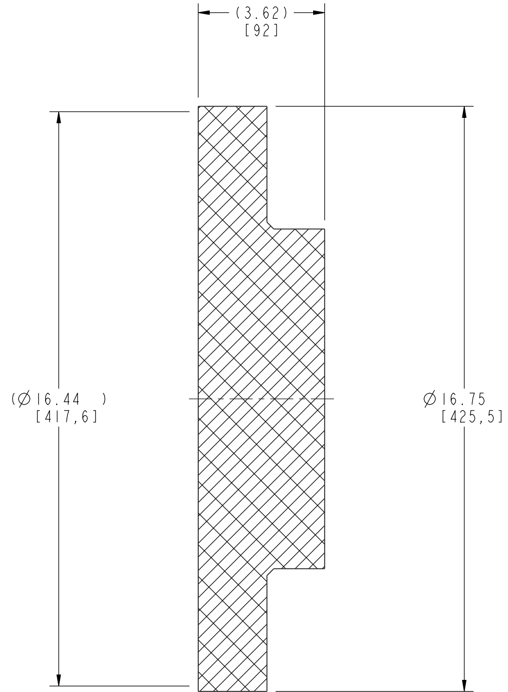
SECTION A-A
